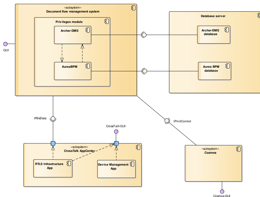
Fig. 2. Logical architecture of the privileges module Rys. 2. Architektura logiczna modułu przywilejów
