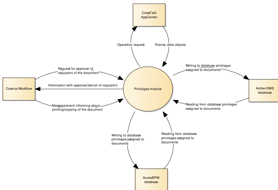
Fig. 1. Perspective of the module of privileges Rys. 1. Perspektywy modułu przywilejów
